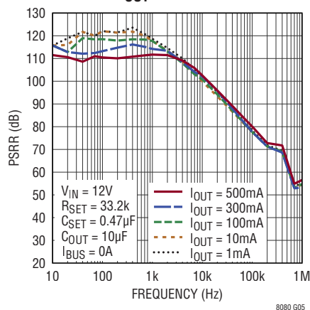
PSRR vs I_{\text{OUT}}
