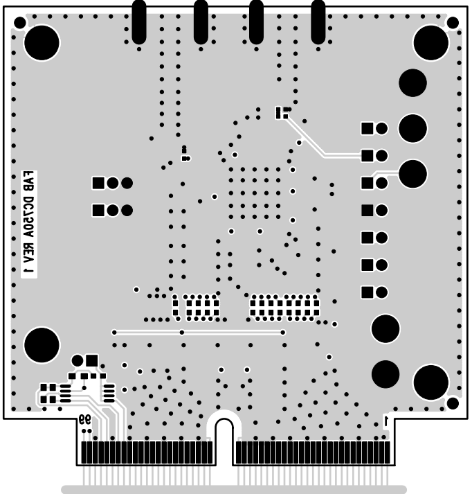
Layer 4 Bottom Side
