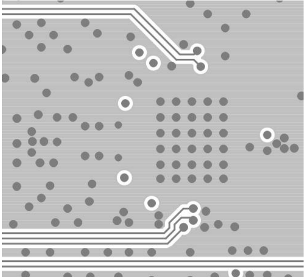
Inner Layer 3
