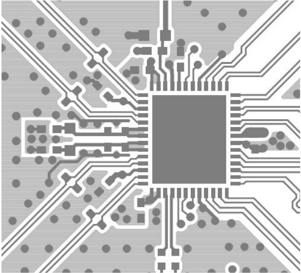
Top Side
