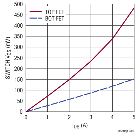
Switch V_{DS}
