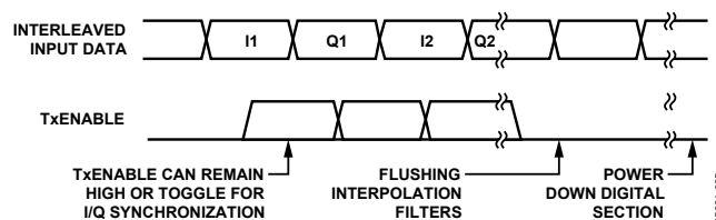
Figure 91. TXENABLE Function
