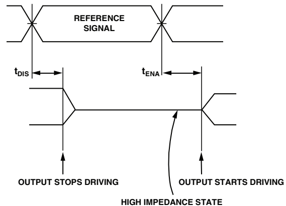
Figure 28. Output Enable/Disable
